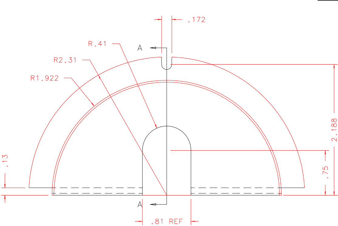
FRONT:SCALE 1:1
