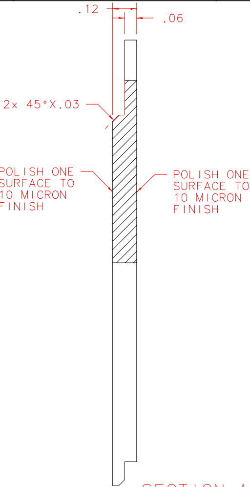
SECTION A-A SCALE 2:1
