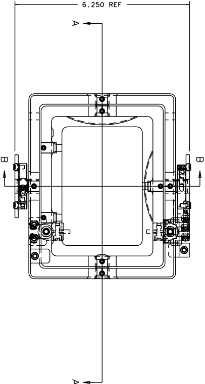
FRONT: SCALE 1 : 2
