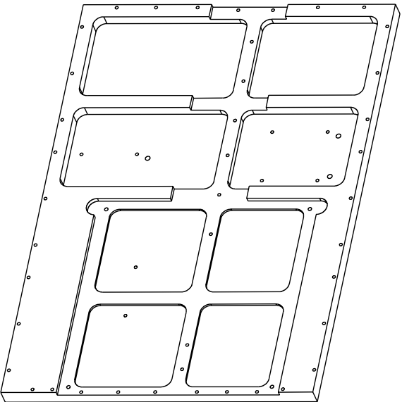
VIEW8: SCALE 1:4
