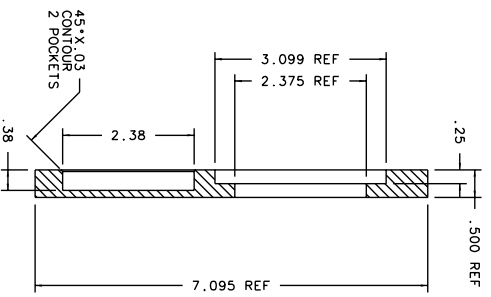
SECTION A-A: SCALE 1:2
